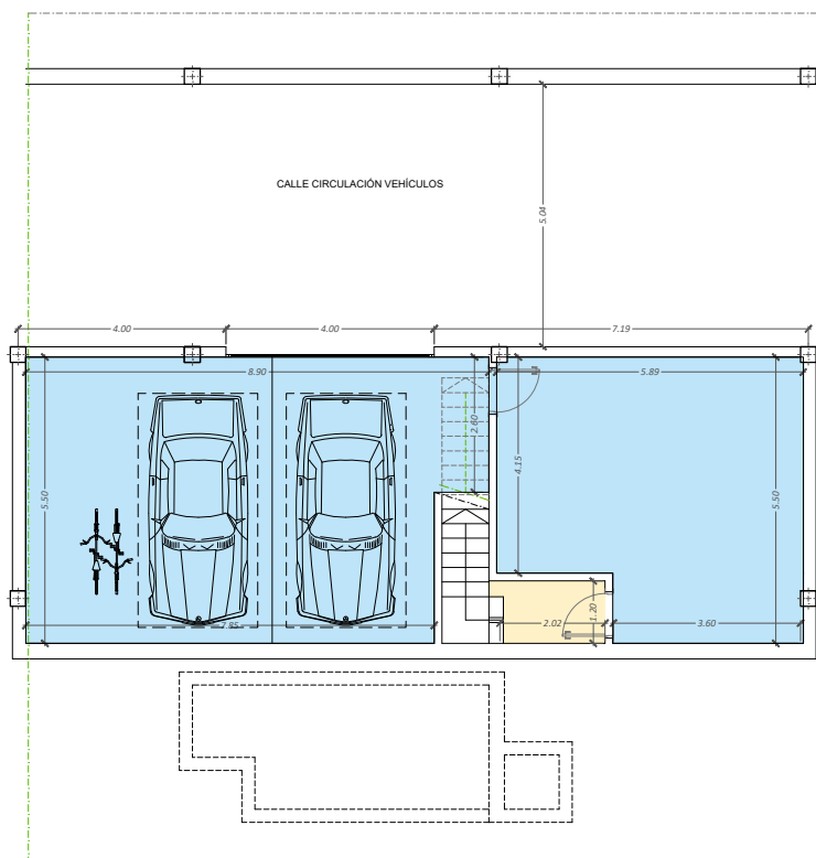
PLANTA SOTANO
