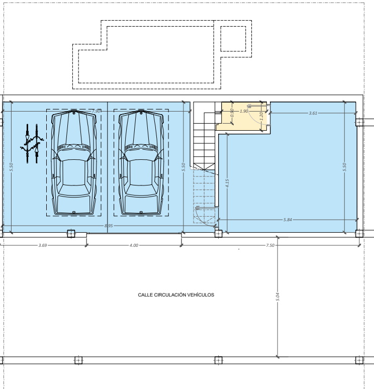
PLANTA SOTANO
