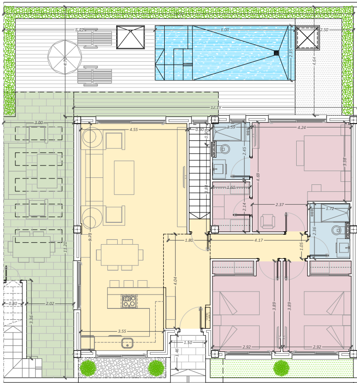
PLANTA BAJA
