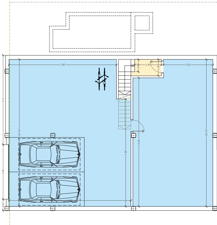
PLANTA BAJA
