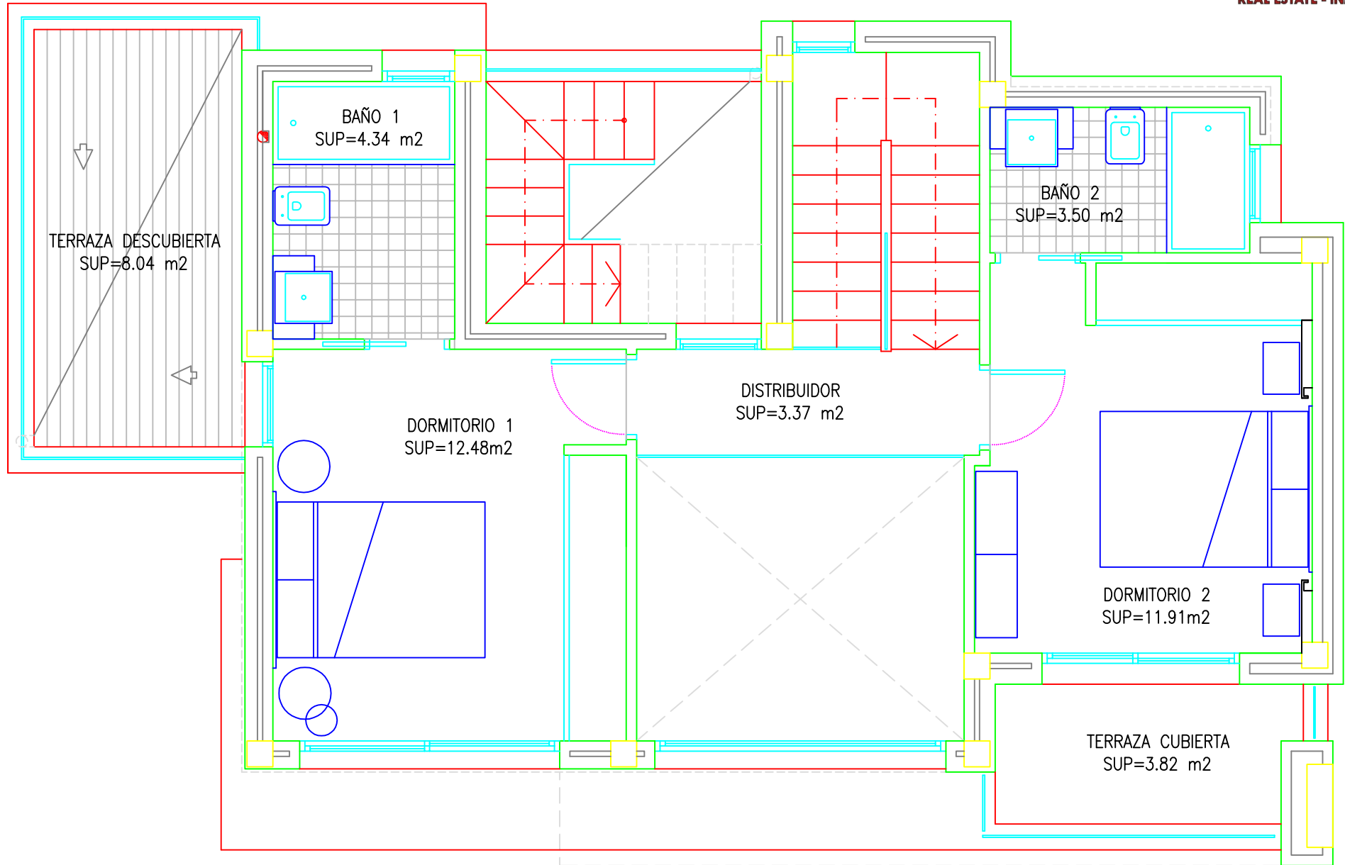
PLANTA PRIMERA
