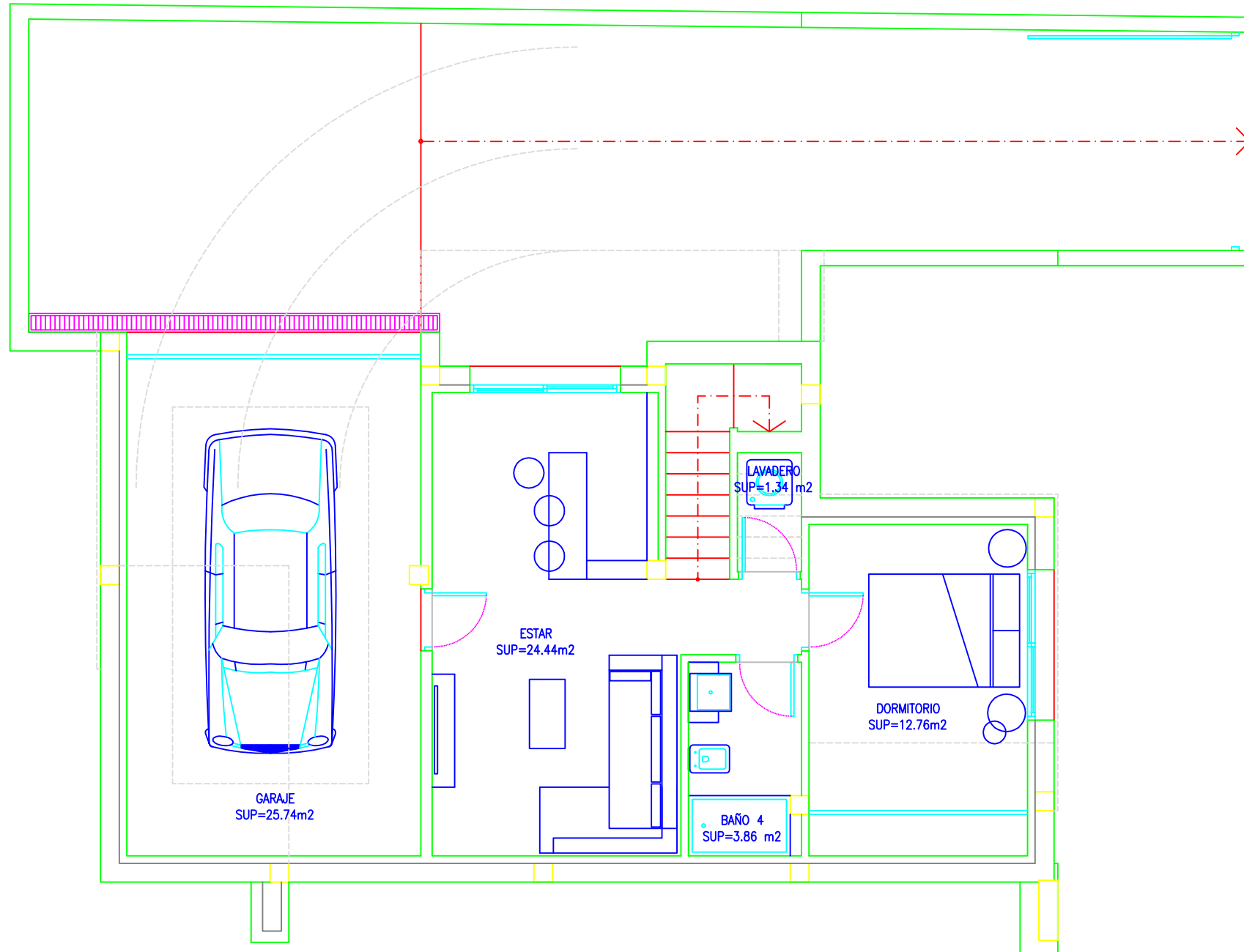
PLANTA SÓTANO
